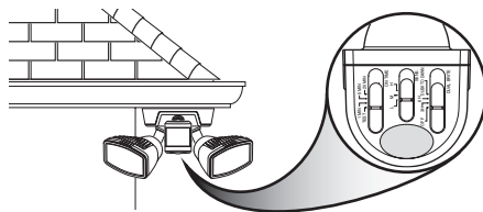
Montage sous avant-toit
